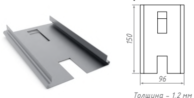
Удлинитель кронштейна
