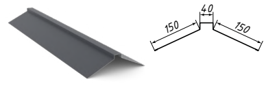
Конёк плоский
