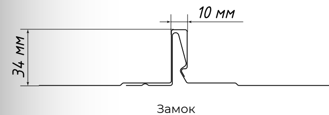
Замок
