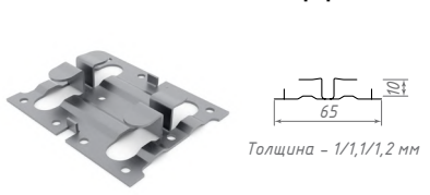
Кляммер рядовой
