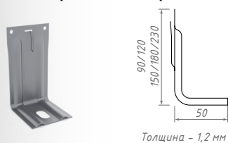
Крепёжный кронштейн
